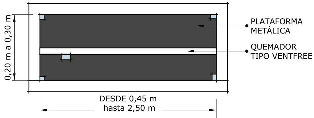
VISTA SUPERIOR
