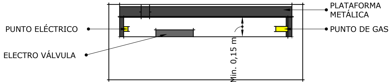
CORTE FRONTAL
